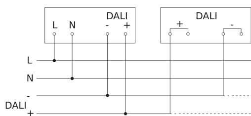
Diagrama electrónico interconexión DALI-2 APC con DALI-2 IPD
