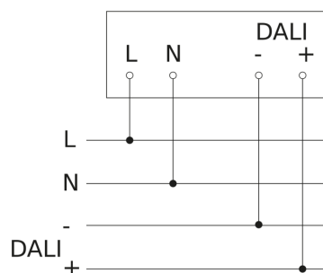
Diagrama electrónico maestro
